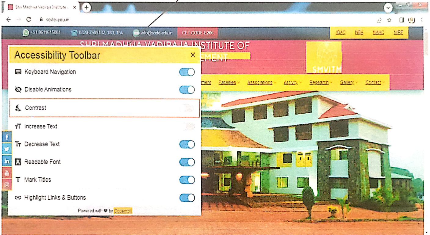
Tool Bar
